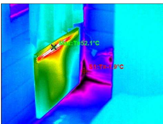
Seinän nurkkarakenteessa paha ilmavuoto, nurkassa pakkasta -1,9 °C
