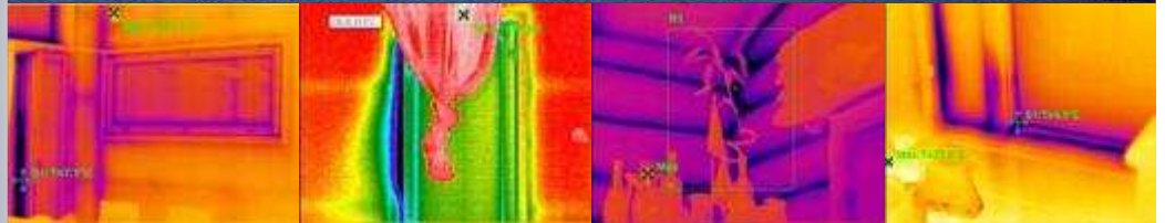
Ikkunaelementin ja karmin välinen ilmavuoto
